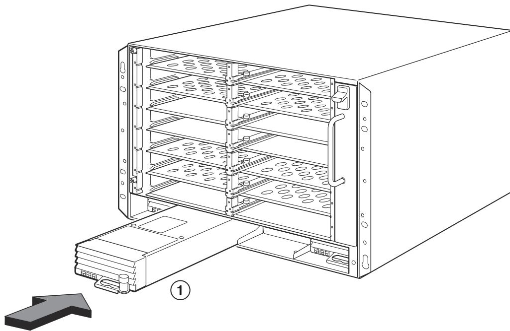
GAMBAR 86 Memasang catu daya di dalam sasis 8 slot
